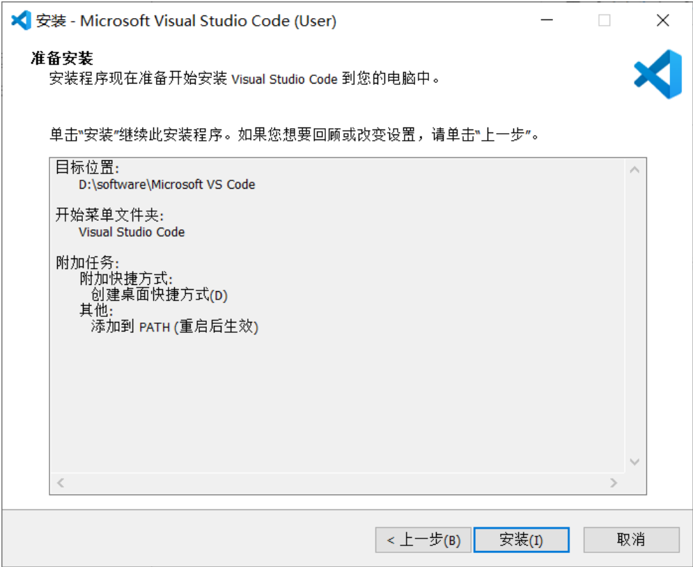
图 2.39 安装 VSCode
