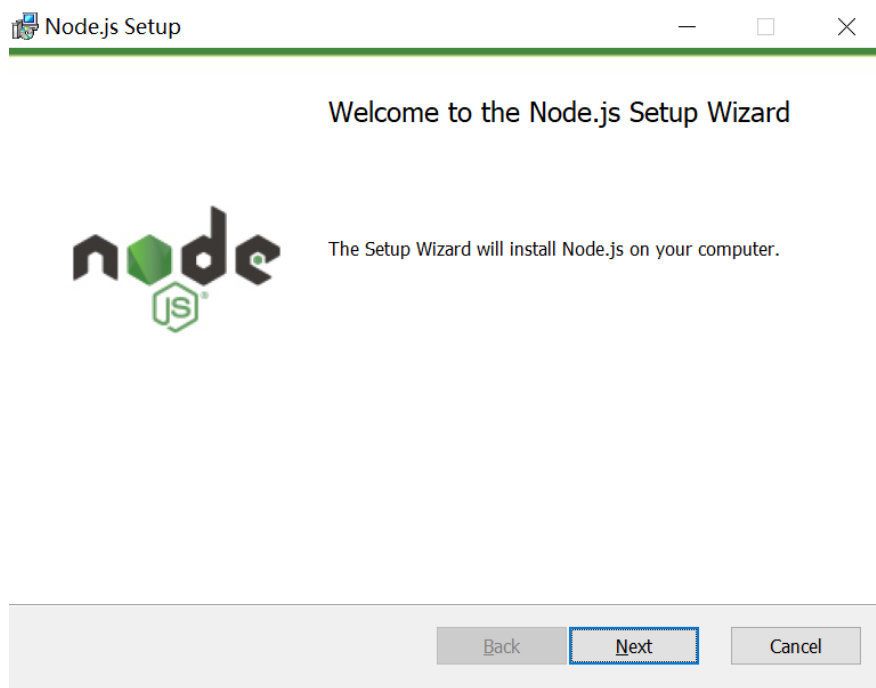
图 2.57 Node.js 安装
