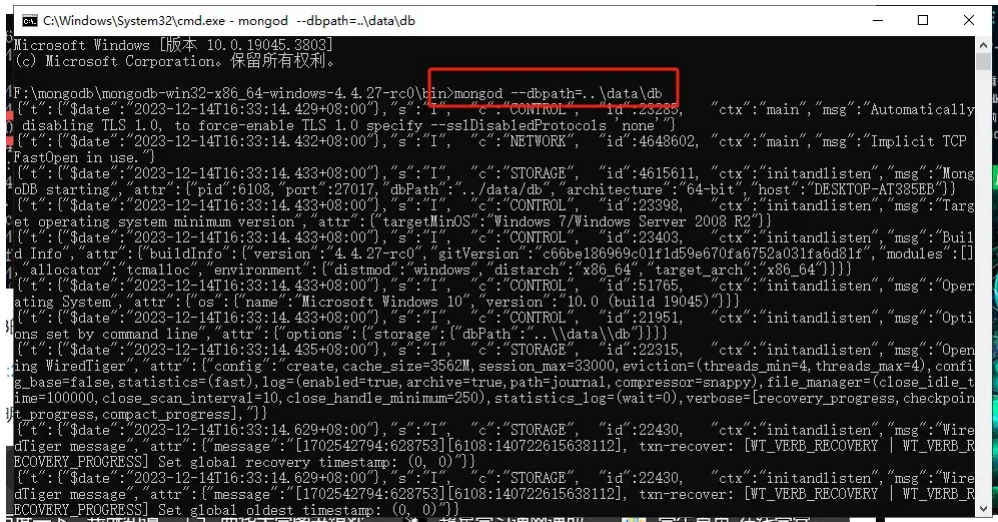
图 2.23 Mongodb 启动
