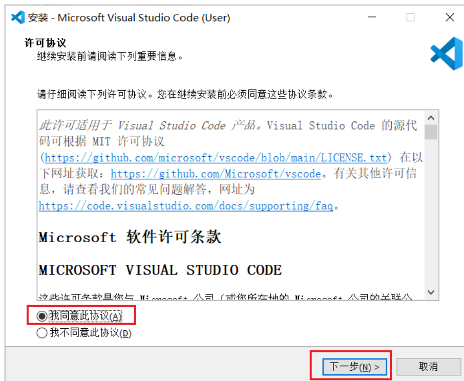
图 2.37 安装 VSCode
