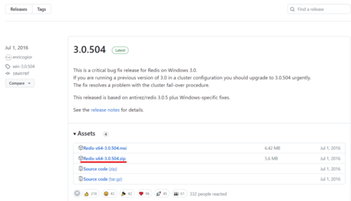
图 2.25 Redis 下载
