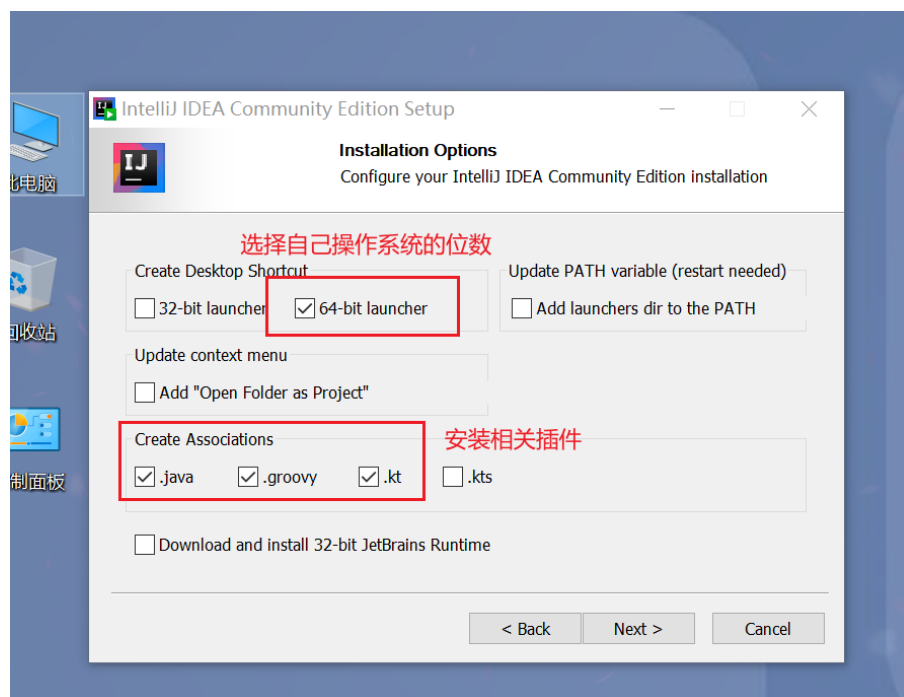
图 2.33 配置桌面设置与相关插件
