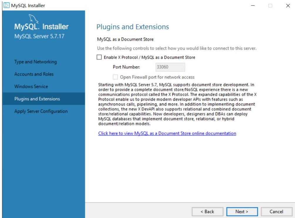
图 2.9 插件与扩展配置
