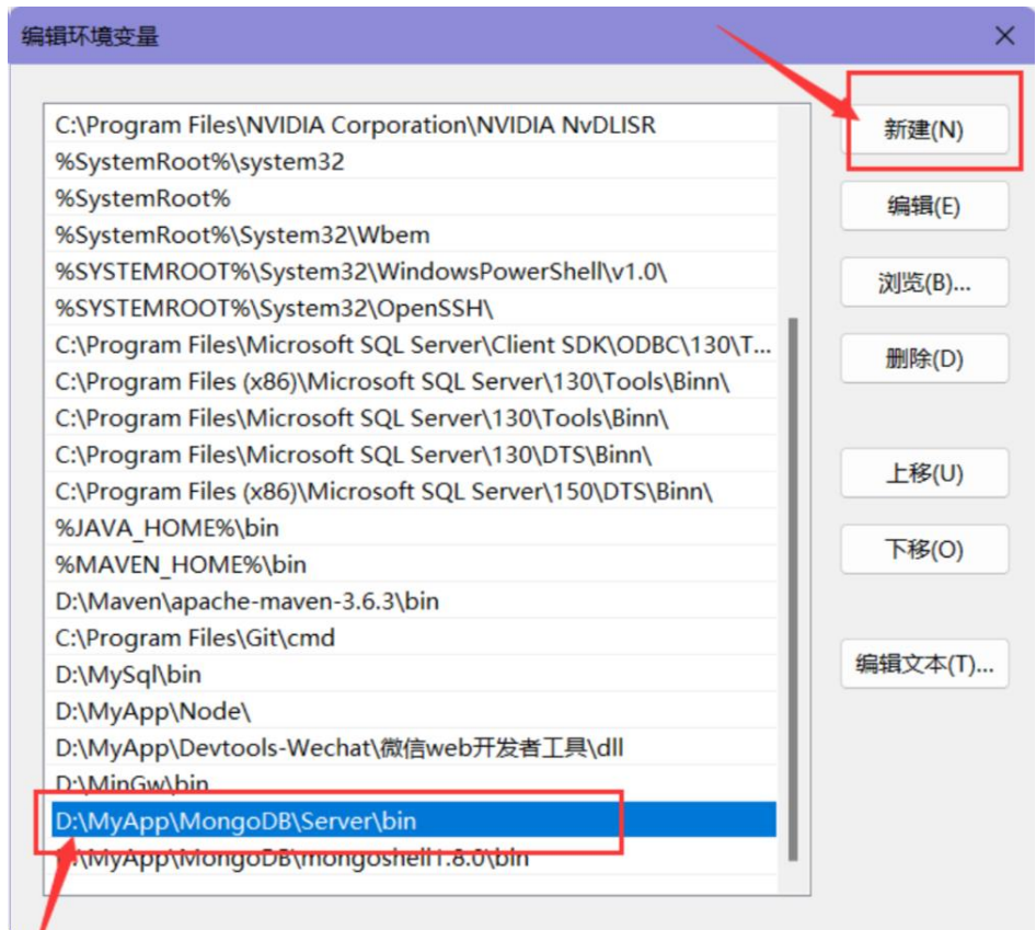
图 2.21 环境配置
