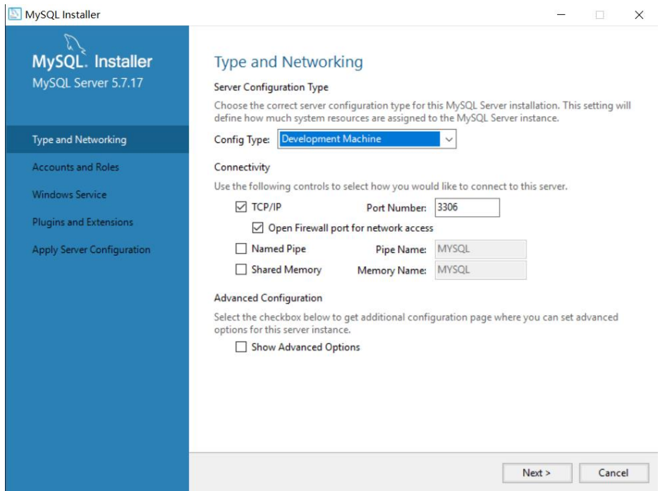
图 2.6 MySQL 配置
