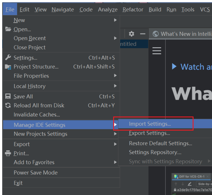
图 2.35 配置 IDEA
