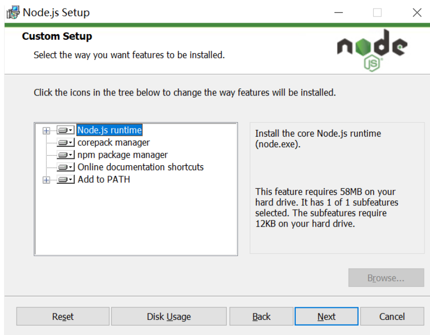
图 2.60 选择 Node.js
